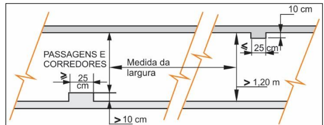
Figura 1: Medida da largura em corredores e passagens
