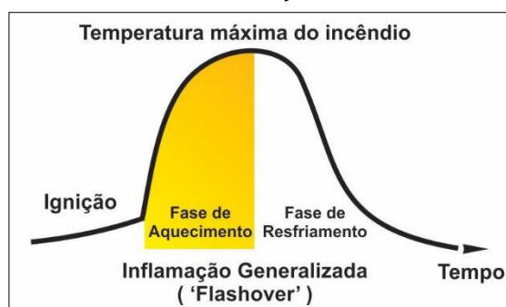
Figura 17: Curva temperatura-tempo de um incêndio
