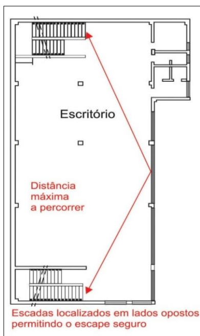
Figura 37: Localização e caminhamento para acesso a uma escada.
