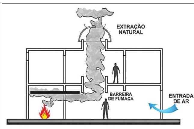
Figura 25: Extração de fumaça de áticos.
