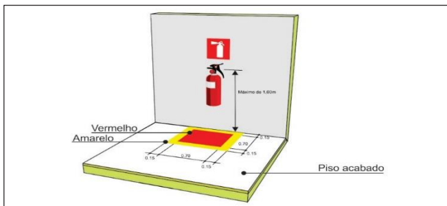
Figura 53: Detalhe de instalação de extintores em áreas sujeitas à obstrução.
